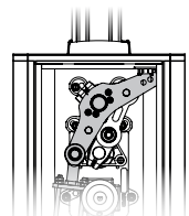
Mástil en vertical (muelle recogido)
